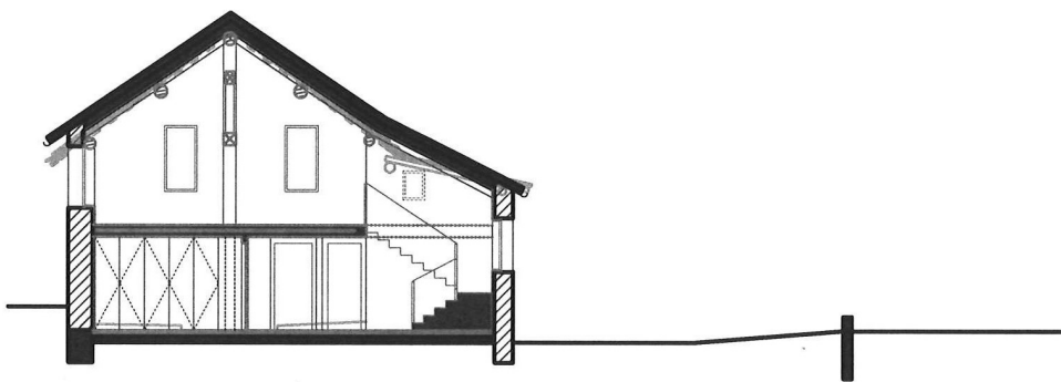
SEZIONE AA
