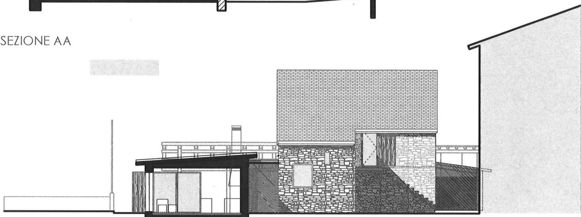
FACCIATA SUD
